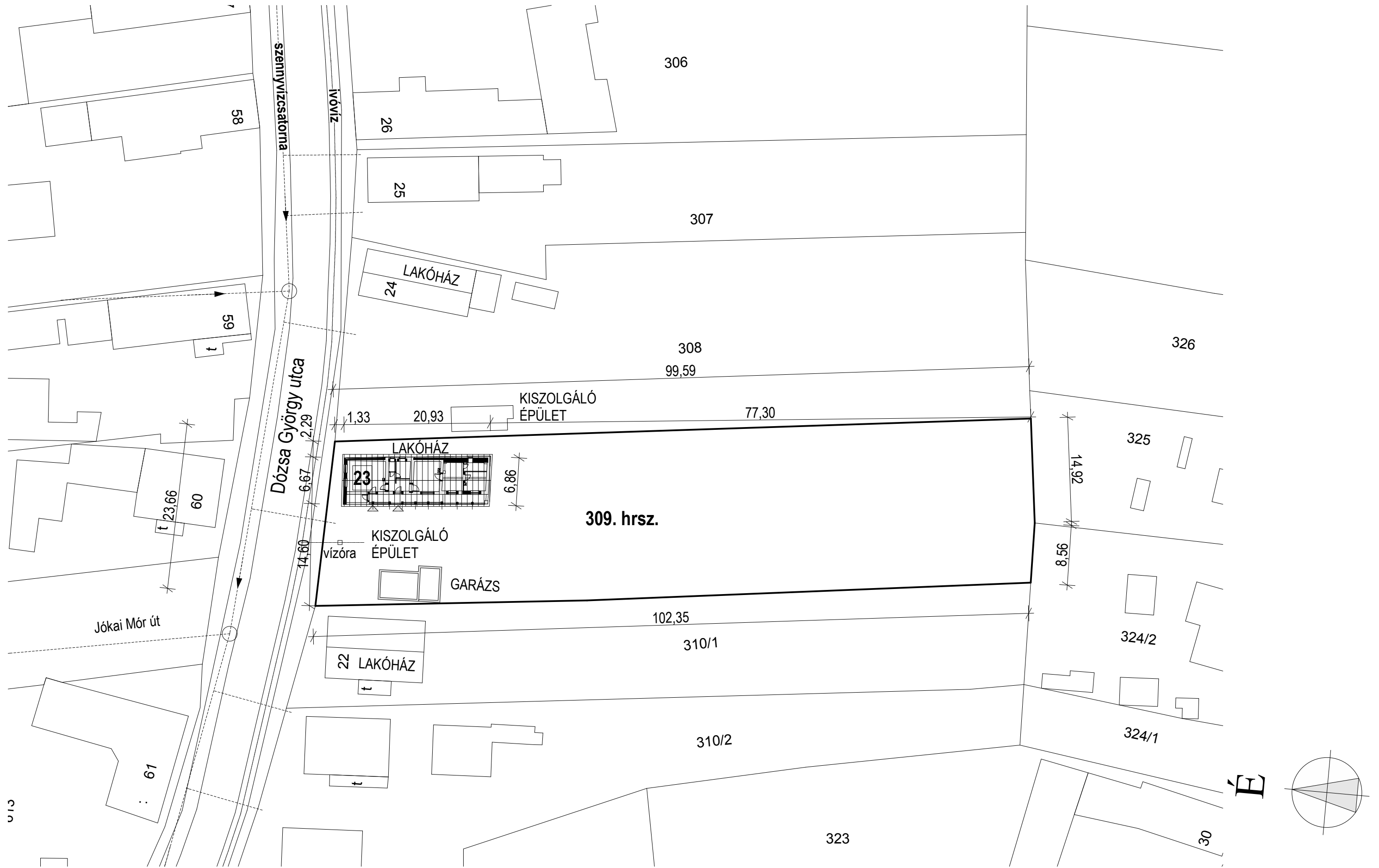
HELYSÍNRAJZ M 1:500
