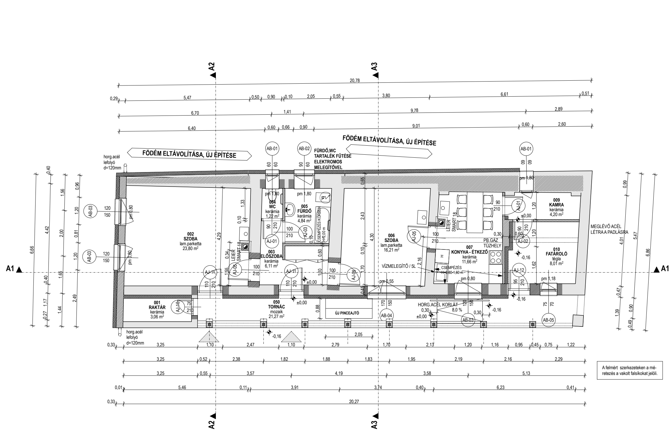
ALAPRAJZ M 1:100 HELYISÉGLISTA
